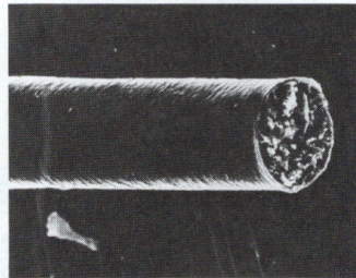
No 5 カット不良による損傷です。毛先にコルテックス(皮質)の繊維状細胞が露出しています。
