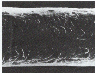
No 4 キューティクルがほとんどはく離し、コルテックス(皮質)が露出しています。
